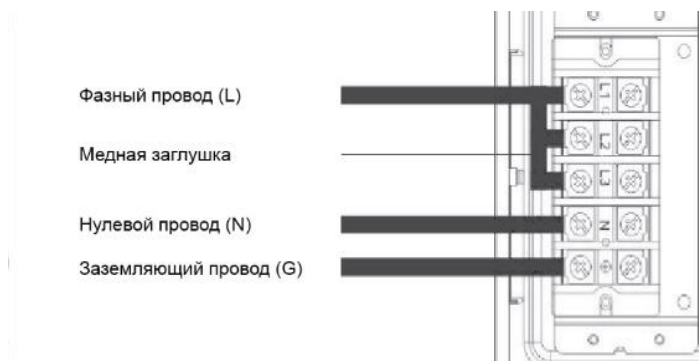
Рис. 8. Однофазное подключение прибора – зеркальный порядок
