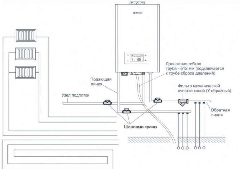
Рис. 5. Схема подключения труб
